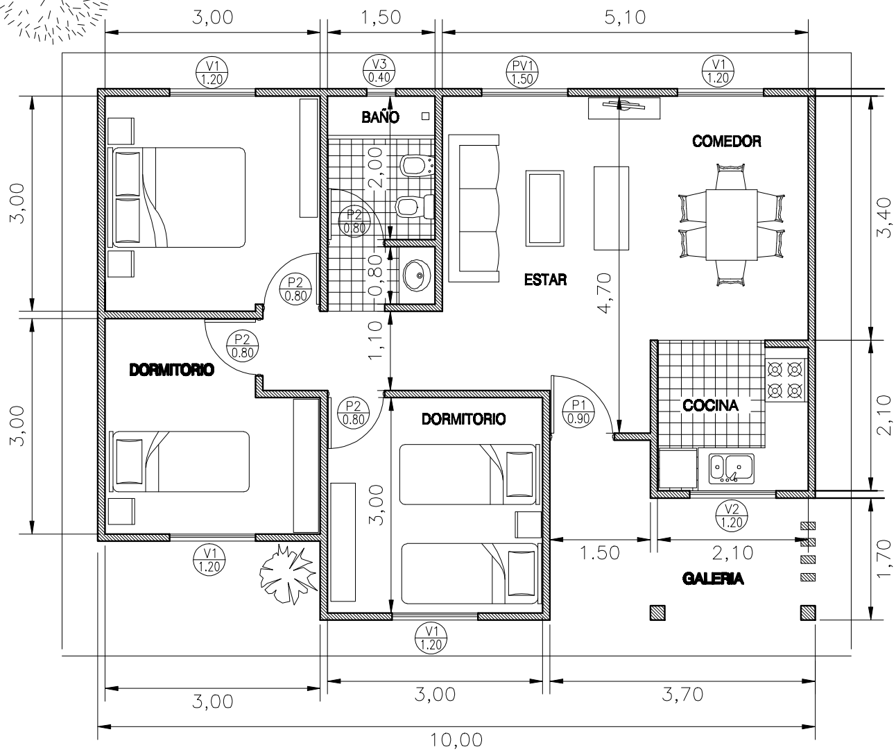
VIVIENDA 3 DORMITORIOS
