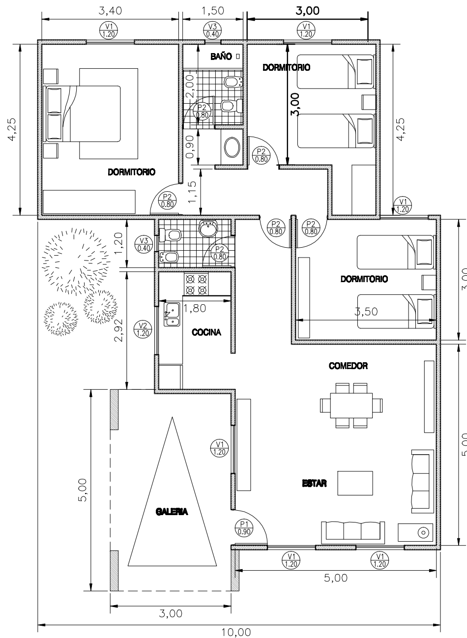
VIVIENDA ESTANDAR 3 DORMITORIOS
