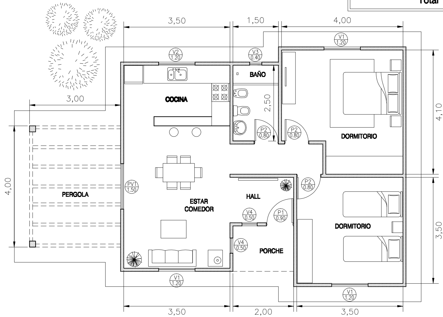
VIVIENDA ESTANDAR 2 DORMITORIOS
